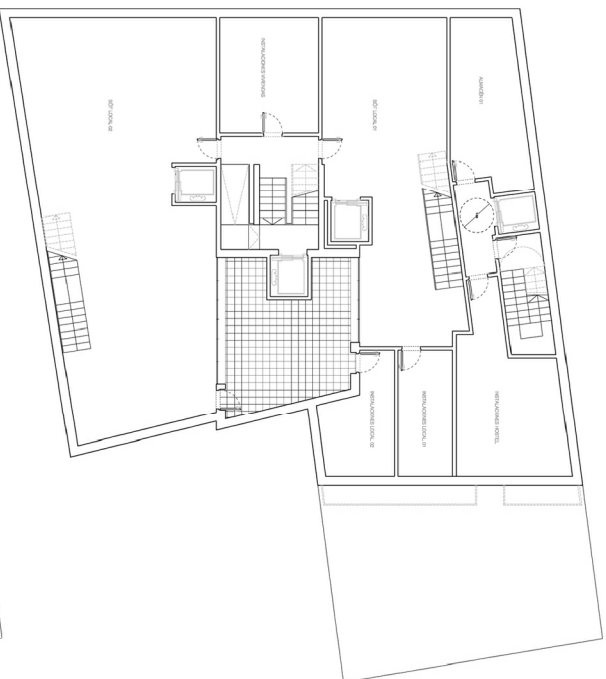
PLANTA SÓTANO
