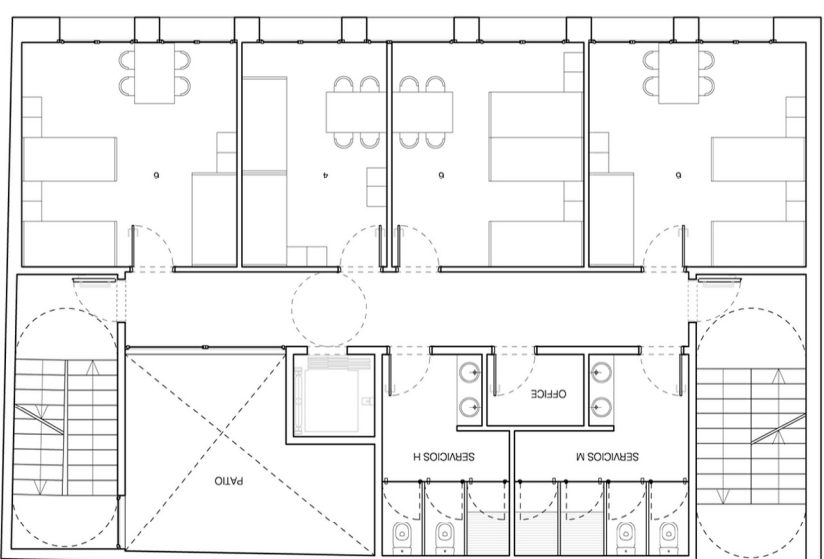
C PLANTA TIPO (4 habitaciones)
