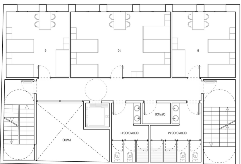
B PLANTA TIPO (3 habitaciones)
