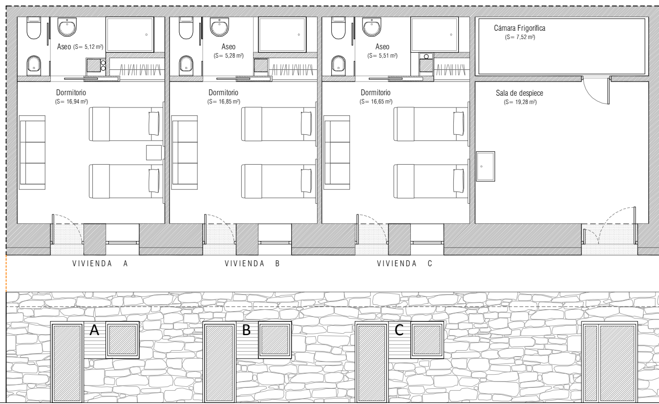
planta baja (estado reformado v.1)
