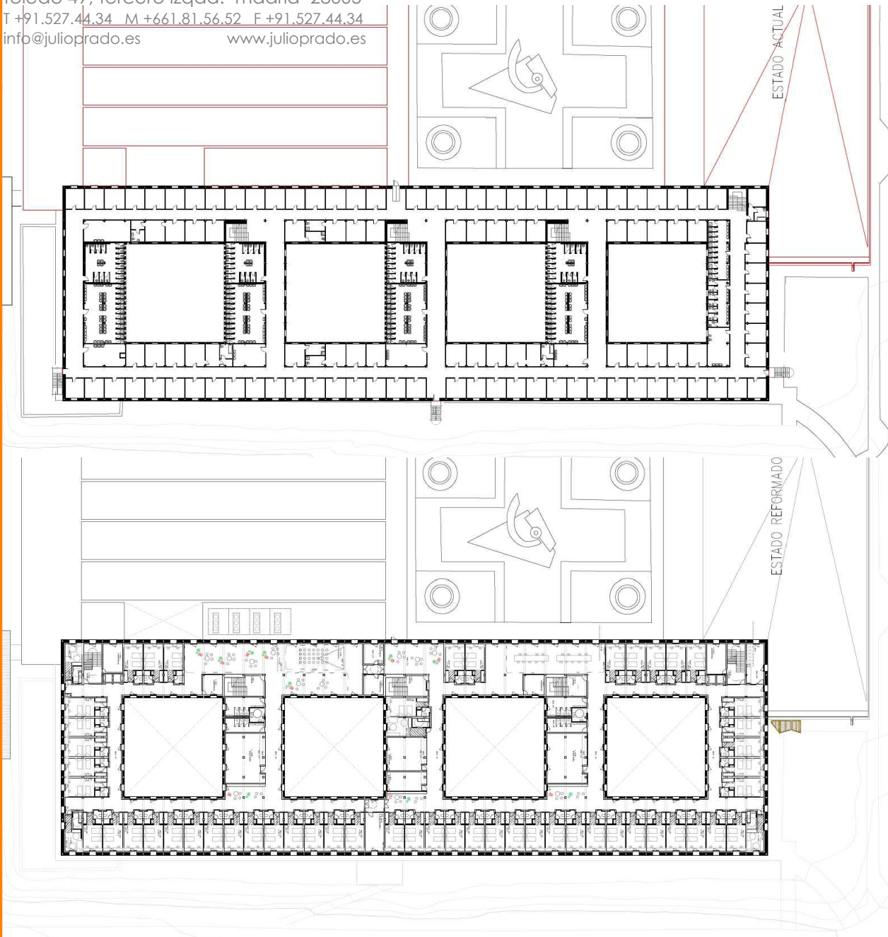
PLANTA 1-2 ESTADO ACTUAL
